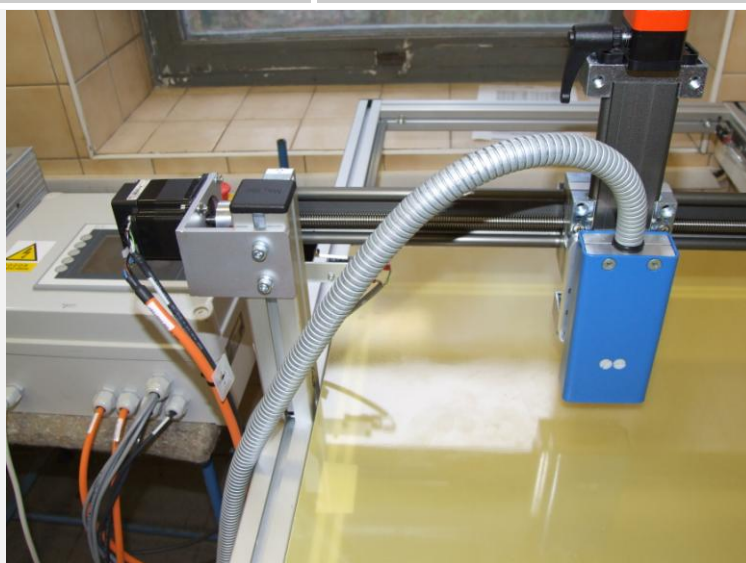
Zvýšení povrchové energie v oblasti aktivace tryskou (>38 mN/m)
